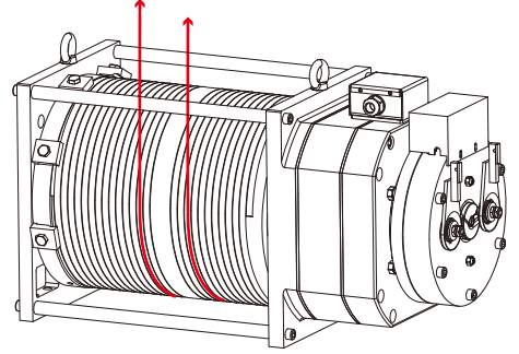
Alttan Montaj, halatlar yukarıya doğru çekilir Bottom Installation, ropes out upward
