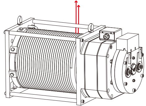
Alttan Montaj, halatlar yukarıya doğru çekilir Bottom Installation, ropes out upward
