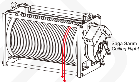
Üstten Montaj, halatlar aşağıya doğru çekilir Top Installation, ropes out downward
